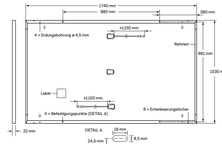
Abb. 1: Außenmaße (in mm) und Komponenten für Q.PEAK DUO-G8, Q.PEAK DUO BLK-G8, Q.PEAK DUO-G8+ und Q.PEAK DUO BLK-G8+
